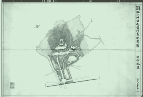
官幣大社近江神宮造営計画配置図(建物配置)
