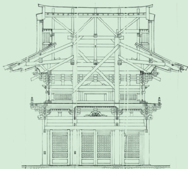
楼門回廊桁行断面詳細図
